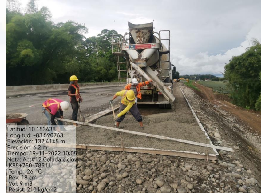
Ciclovía del Km 85+750 al 85+785, Lado izquierdo
