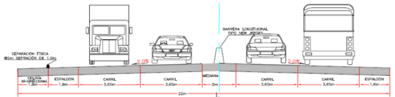
SECCIÓN TÍPICA 3
