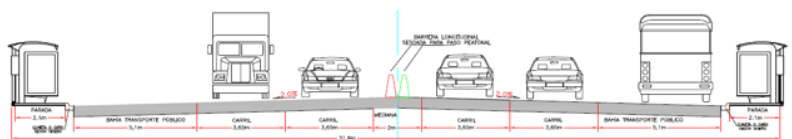
SECCIÓN TÍPICA 4
